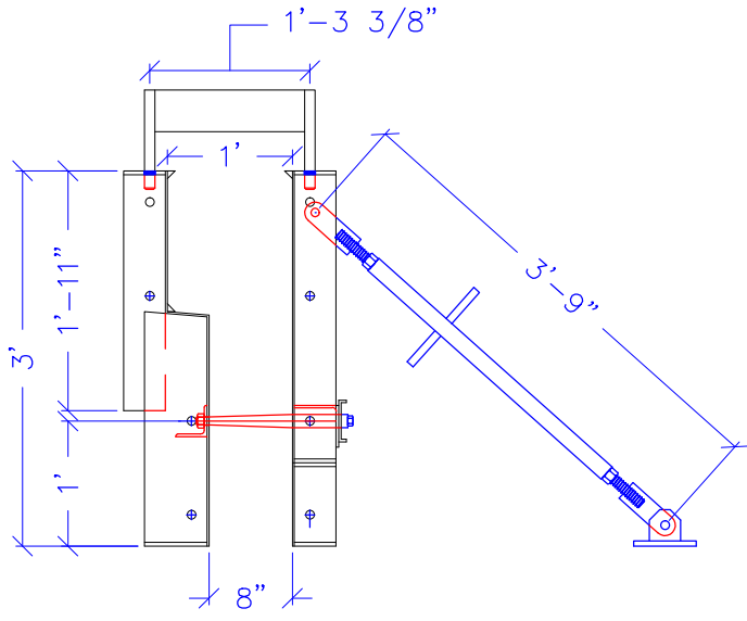
END ELEVATION
