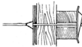
Snapties
